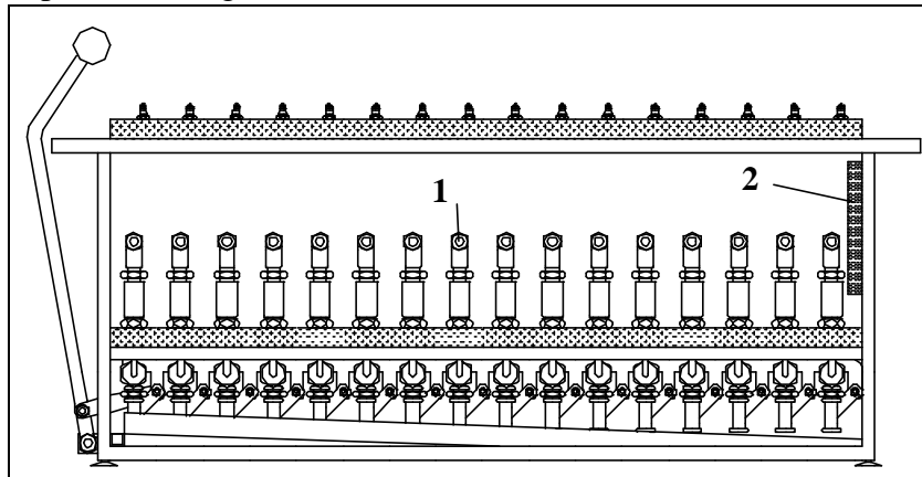
Fig. 3 – Vista posteriore del banco di misura: 1. sensore; 2. contattiera.
